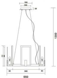
Габаритные размеры
