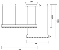
Габаритные размеры
